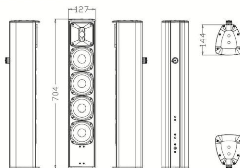
CL4025BT/CL4025WT
